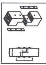
Detalhe das emendas dos Pilares S/Escala
